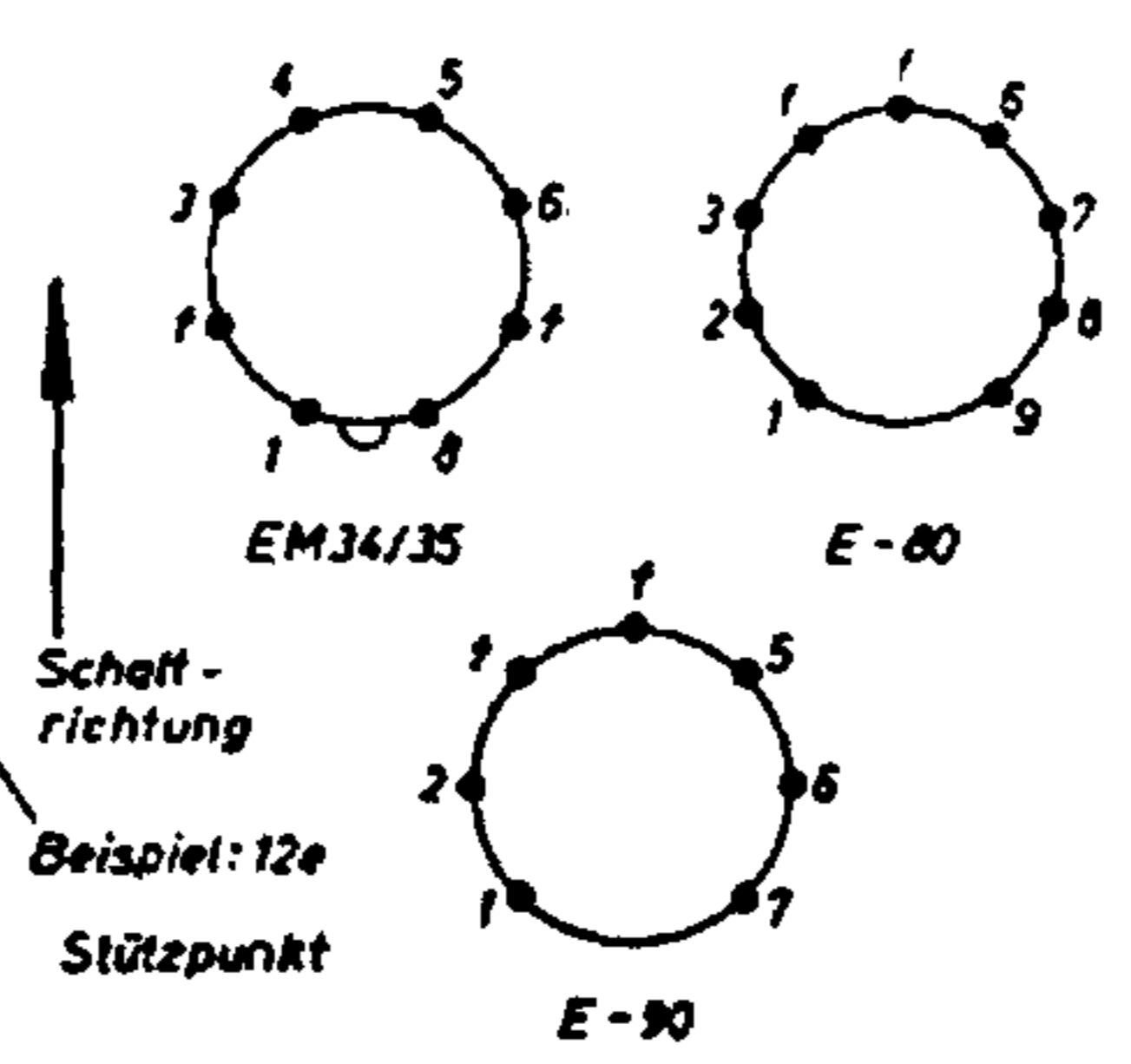
Schalt-richtung Tasten in Ruhstellung
