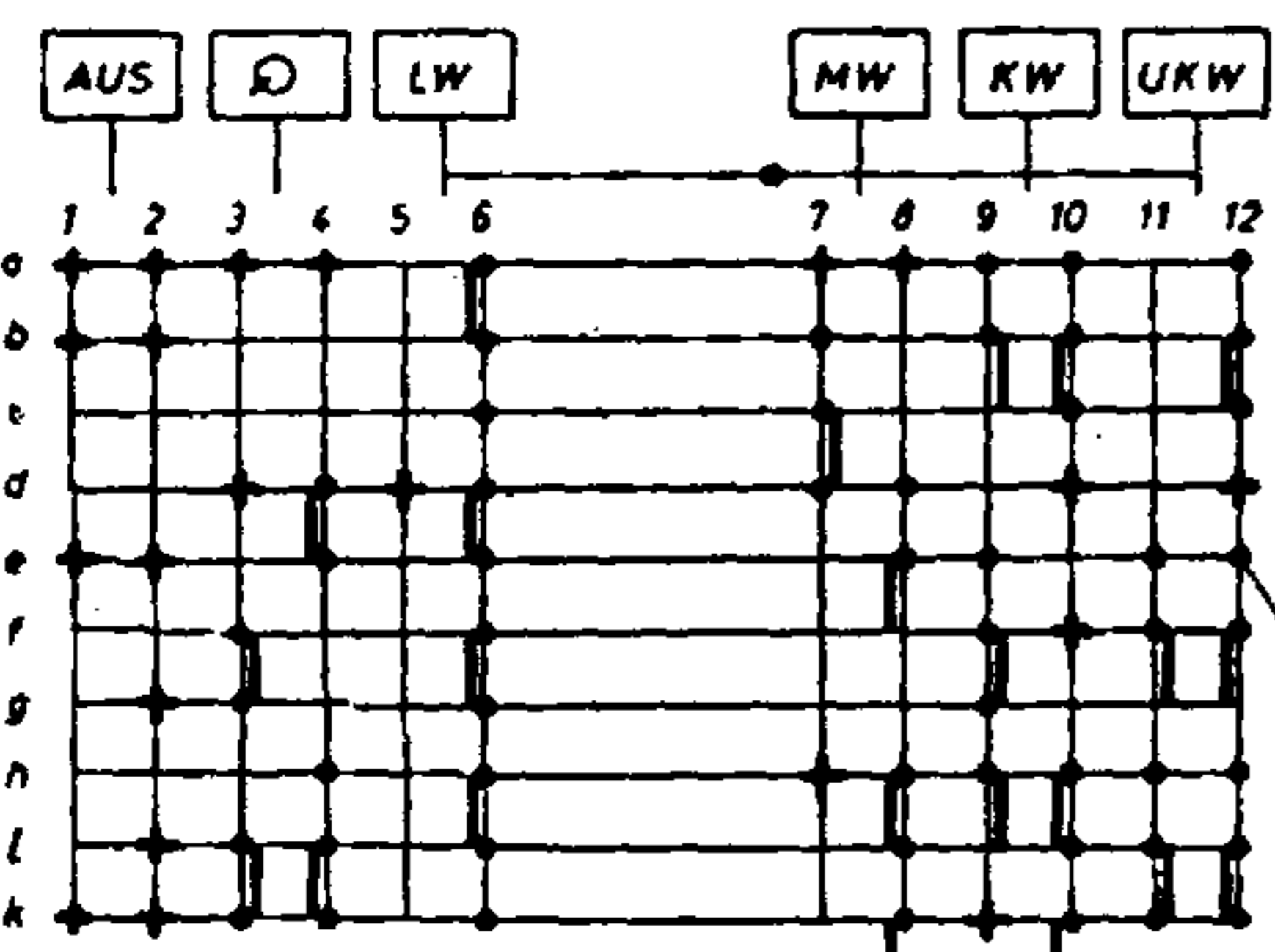
gezeichnete Tastenstellung: Gerät „aus“
